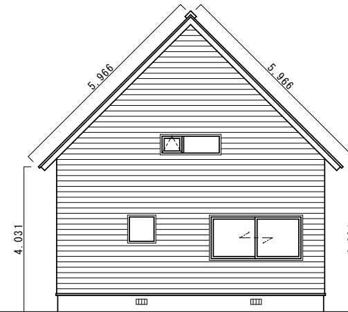
南側立面図
