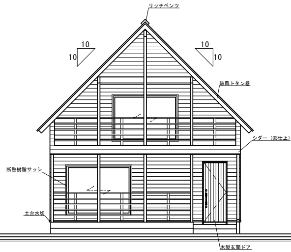
東側立面図
